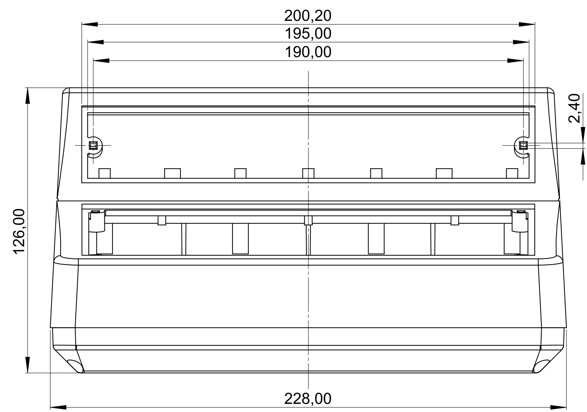
Oberteil Aussenansicht Top part Outside view
