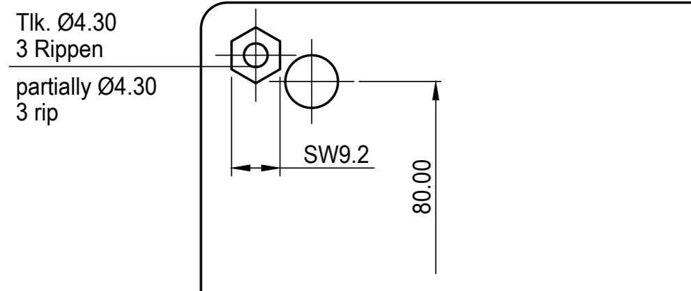
Unterteil Aussenansicht base part outside view
